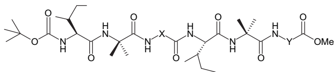
Figure 1. Schematic representation of peptides I–III . Peptide I : X=–CH–CH 2 –CH–(CH 3 ) 2 , Y=–CH–CH 2 –CH–(CH 3 ) 2 ; peptide II : X=–CH–CH 2 –CH–(CH 3 ) 2 , Y=–CH–CH 2 –Ph; peptide III : X=–CH–CH 2 –Ph, Y=–CH–CH 2 –CH–(CH 3 ) 2 .
